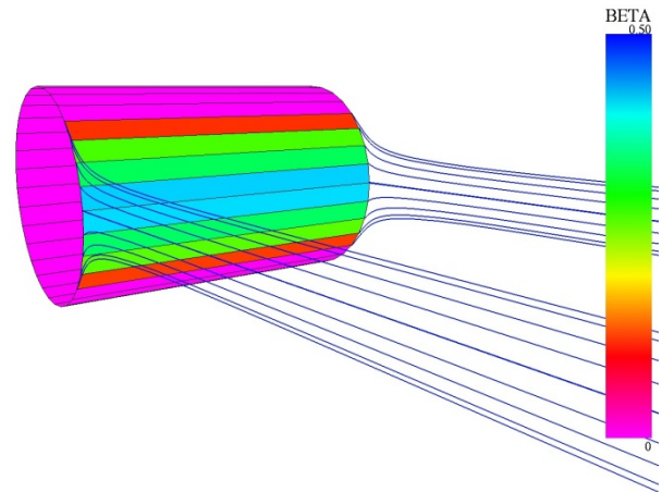
Droplet Trajectories
